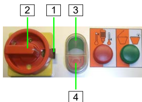
Abb. 74: Maschine wieder einschalten
