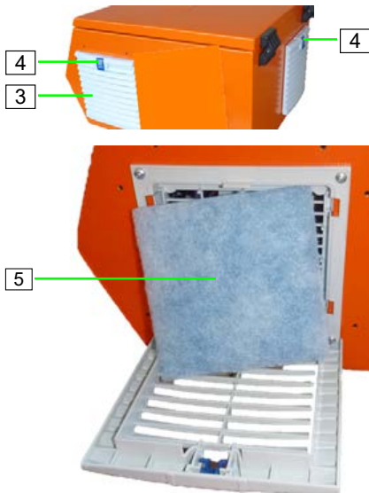
Abb. 79: Filtermatte reinigen
