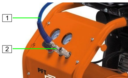
Abb. 31: Luftschlauch anschließen
