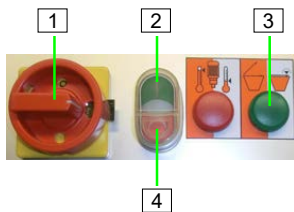
Abb. 38: Maschine einschalten
