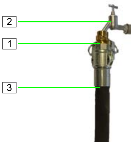
Abb. 26: Mörtelschläuche vorbereiten
