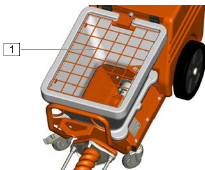
Abb. 19: Gitterabdeckung
