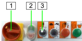
Abb. 69: Rückwärtslauf
