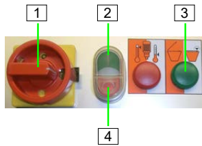
Abb. 29: Einschalten
