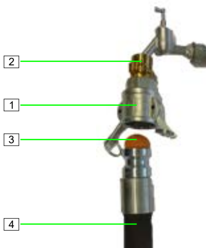
Abb. 62: Mörtelschlauch reinigen
