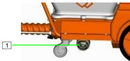
Abb. 30: Reinigungsstutzen öffnen
