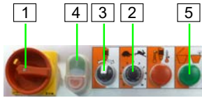
Abb. 37: Maschine einschalten
