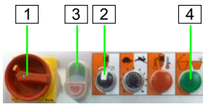
Abb. 57: Maschine nach Stromausfall einschalten
