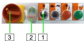
Abb. 52: Maschine ausschalten
