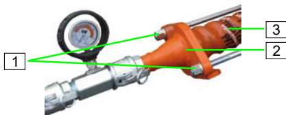
Abb. 80: Pumpeneinheit wechseln
