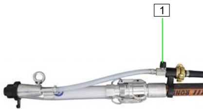
Abb. 46: Lufthahn schließen
