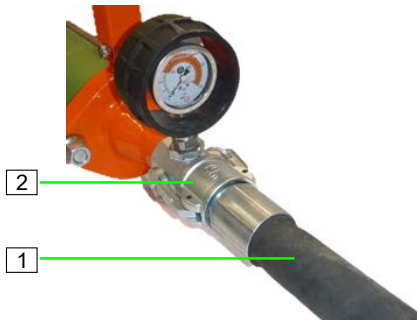
Abb. 27: Mörtelschlauch anschließen
