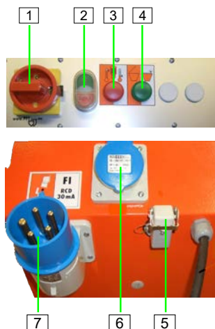
Abb. 11: Baugruppe Schaltschrank
