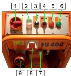
Abb. 8: Baugruppe Schaltschrank
