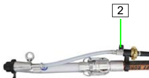
Abb. 45: Lufthahn öffnen
