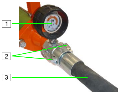
Abb. 61: Mörtelschlauch abkuppeln
